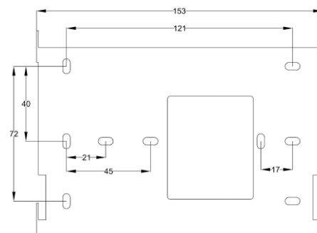
Suport Monitor - Vedere Fata
