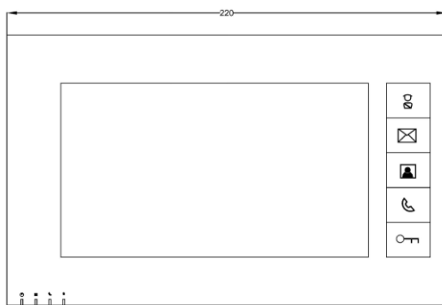
Monitor - Vedere Fata plus conectori
